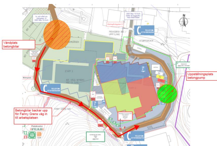
Figur 2. Planerad arbetsgång för större gjutning fredag 15/11 vecka 46.
