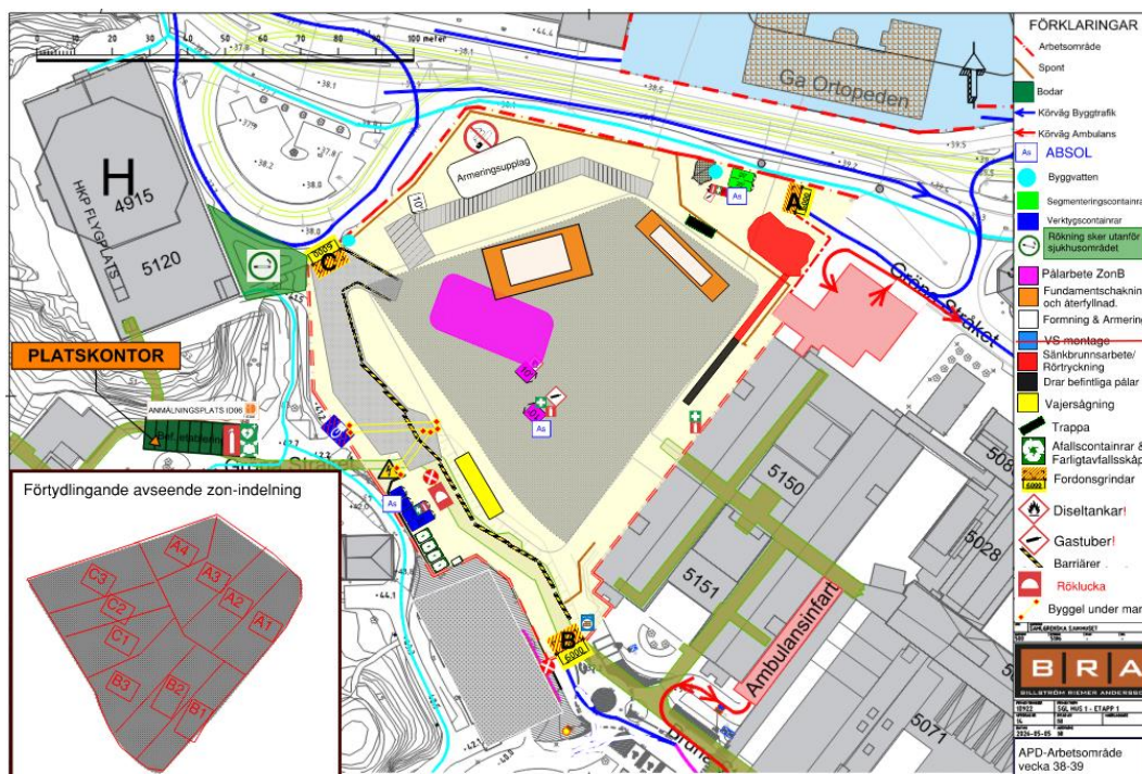
Figur 1 APD-plan (Arbetsplats Dispositions Plan) för byggarbetsområdet.
