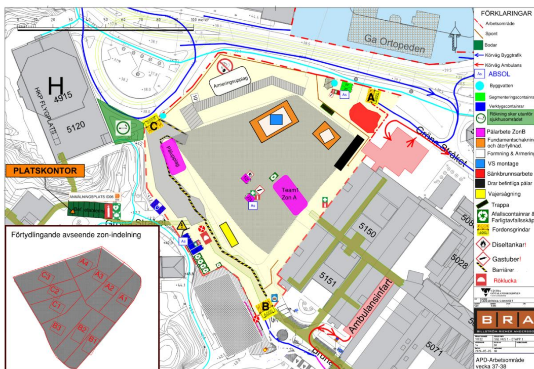
Figur 1 APD-plan (Arbetsplats Dispositions Plan) för byggarbetsområdet.
