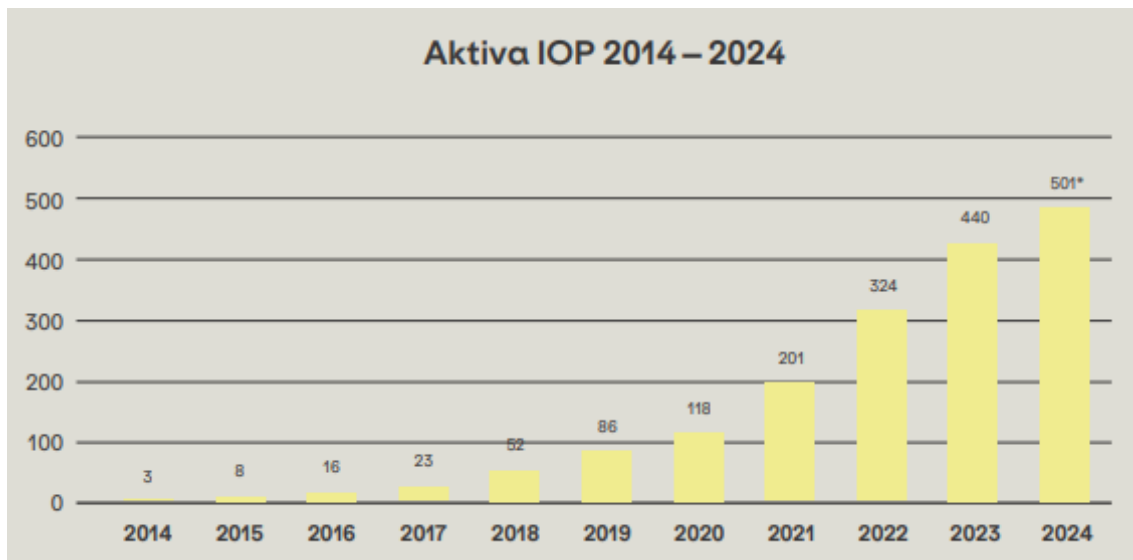
Figur 4: Aktiva IOP 2014-2024
