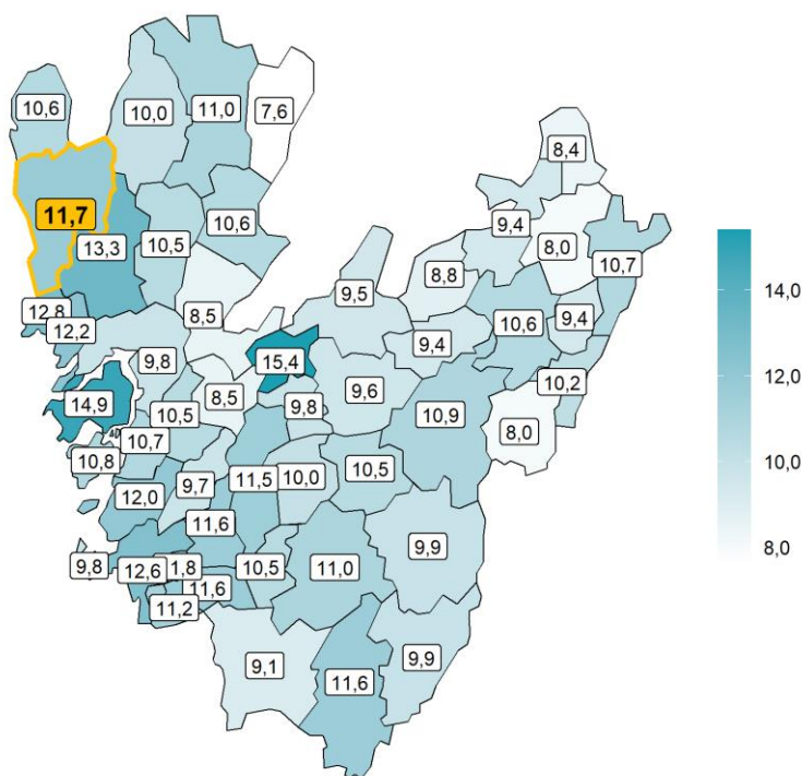
Karta 10. Nyföretagande per 1 000 invånare 2025
