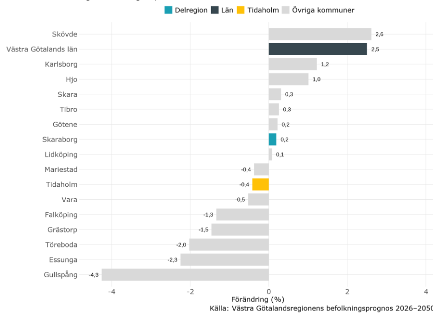
Diagram 5. Befolkningsförändring 2020–2025 i Skaraborg
