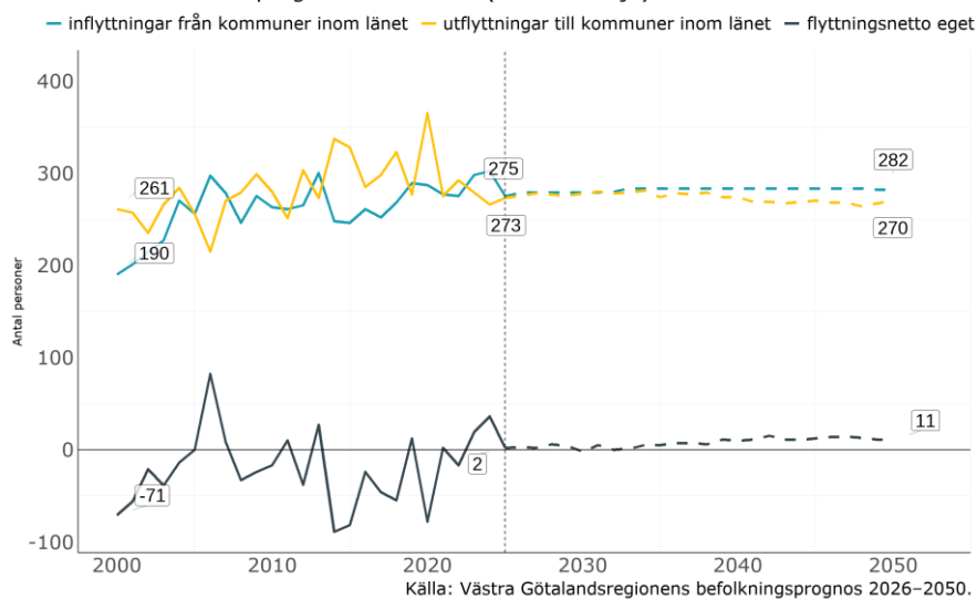
Diagram 13. Flyttningar inom Västra Götaland i Tidaholm
