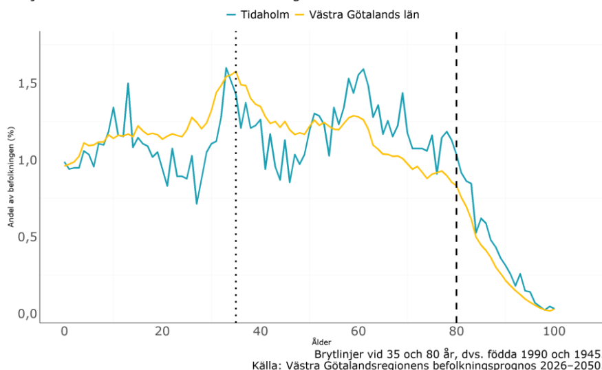
Diagram 4. Åldersstruktur i Tidaholm och Västra Götaland 2025
