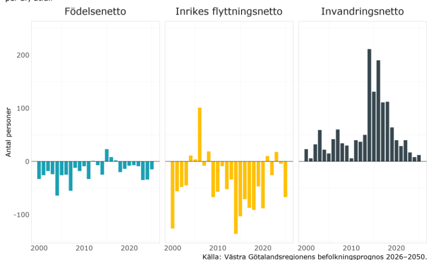
Befolkningsförändringens komponenter i Tidaholm 2000–2025 Födelsenetto, inrikes flyttningsnetto och invandringsnetto per år, utfall
