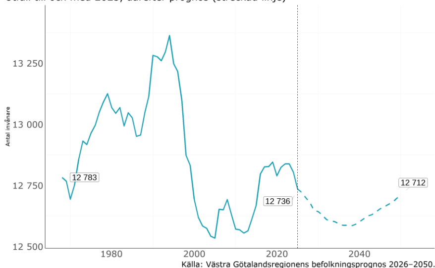
Folkmängd i Tidaholm 1968–2050 Utfall till och med 2025, därefter prognos (streckad linje)
