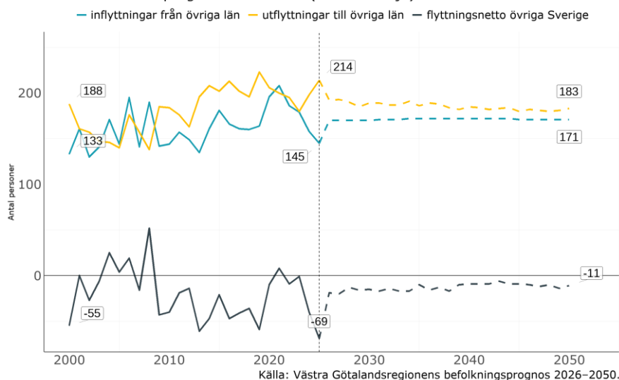
Flyttningar till och från övriga Sverige i Tidaholm Utfall 2000–2025 och prognos 2026–2050 (streckad linje)
