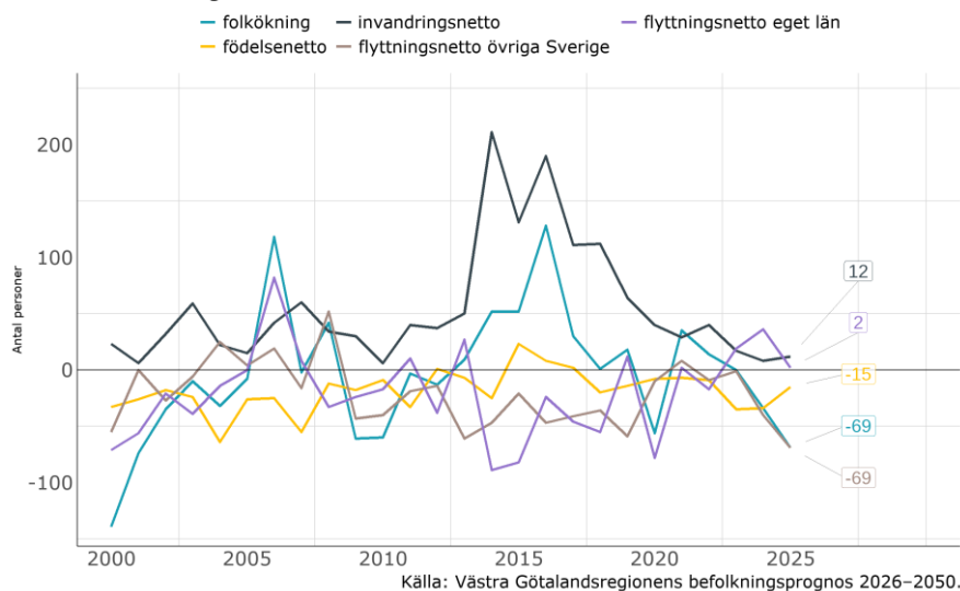
Befolkningsförändringens komponenter i Tidaholm 2000–2025 Historisk utveckling 2000–2025
