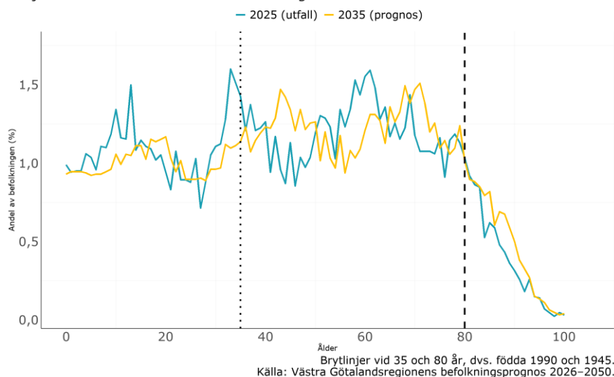
Åldersstruktur i Tidaholm 2025 och enligt prognos 2035 Varje ålders andel av den totala befolkningen
