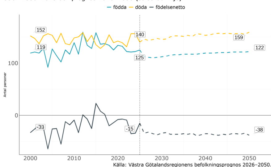
Diagram 15. Födda och döda i Tidaholm
