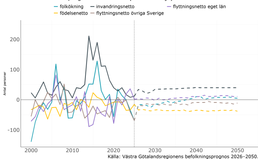
Diagram 6. Befolkningsförändringens komponenter i Tidaholm enligt prognos
