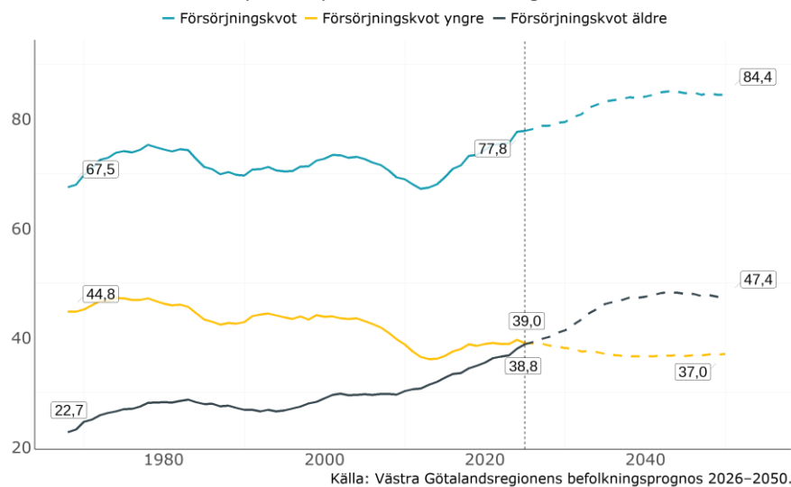
Diagram 11. Demografisk försörjningskvot i Tidaholm
