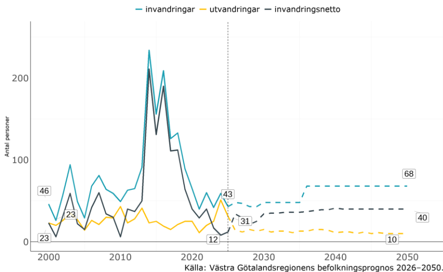
Diagram 14. In- och utvandring i Tidaholm
