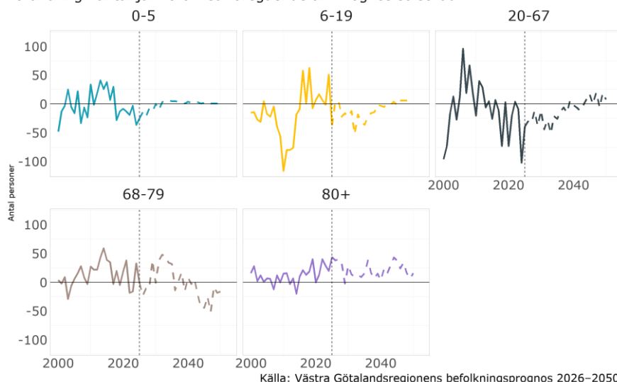
Diagram 9. Årlig förändring per åldersgrupp i Tidaholm
