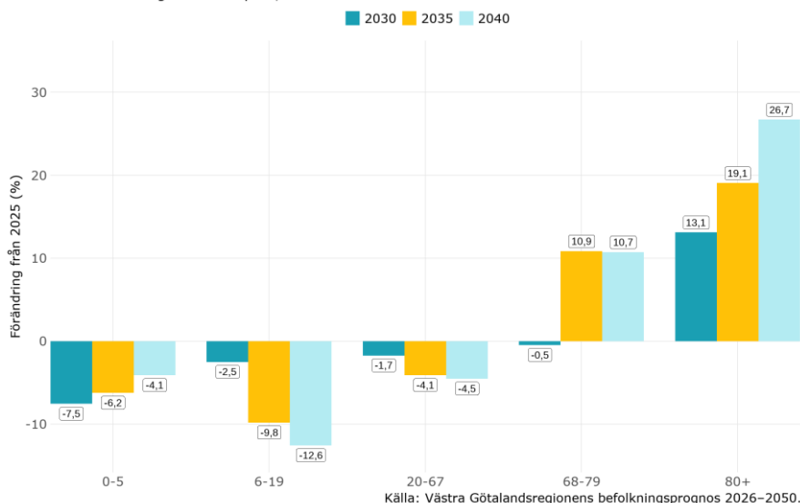
Förändring per åldersgrupp i Tidaholm enligt prognos Procentuell förändring från 2025 på 5, 10 och 15 års sikt
