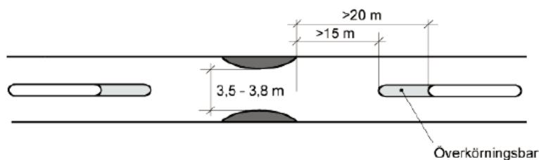
Figur 2.13-8 Exempel på avsmalning med sidohinder och mittrefuger
