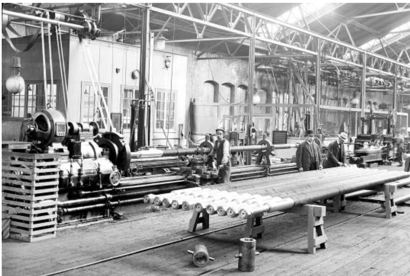
NOHABs industrier i Trollhättan. I den stora svarven tillverkas delar av skruvar till Panamakanalen. Innovatum Bildarkiv
